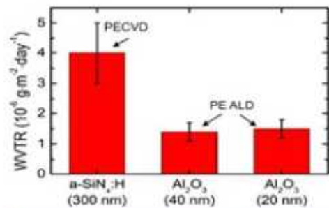
Figure : プラズマALDで、より薄く、より高い防水膜が得られます。
