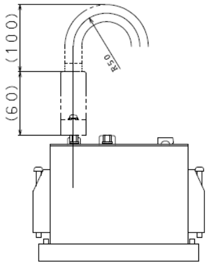
ケーブル取付図詳細
