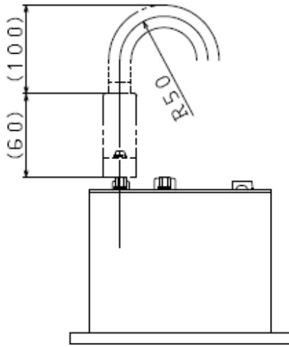
ケーブル取付図詳細
