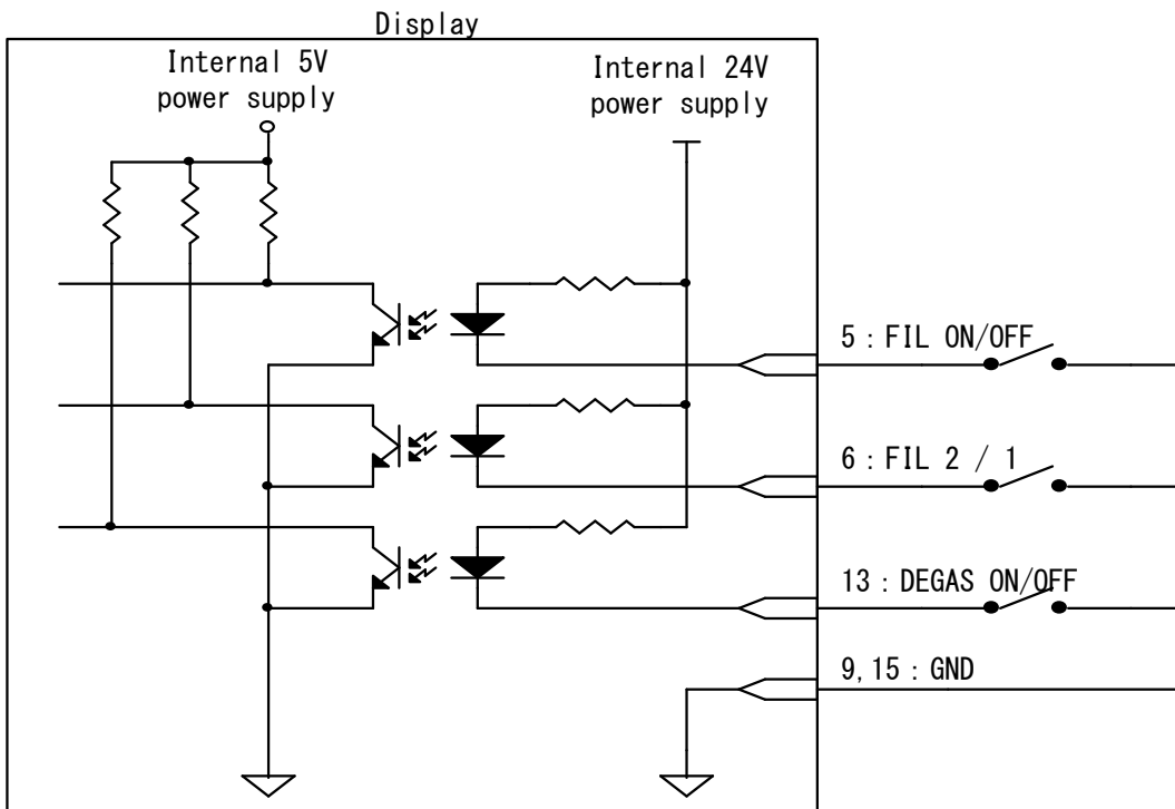
信号入力
