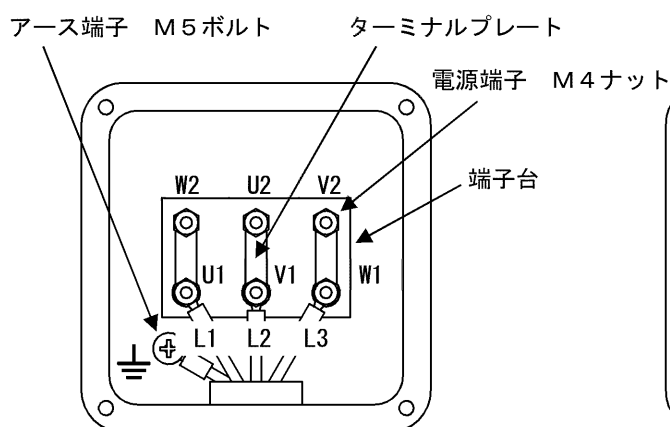
200V級結線 (出荷時結線)
