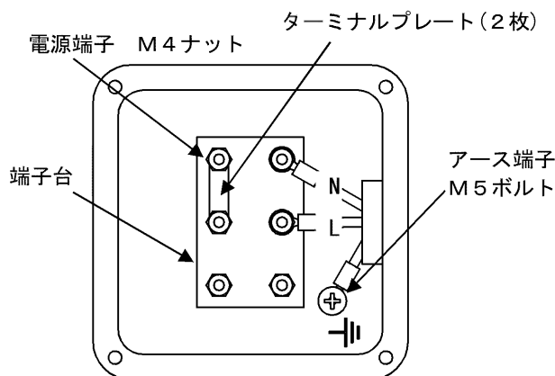
200V級結線 (出荷時結線)
