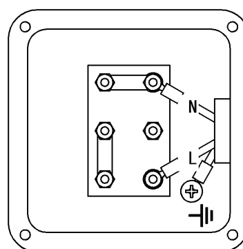
100V級結線
