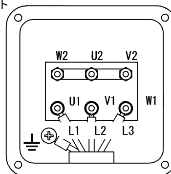
400V級結線
