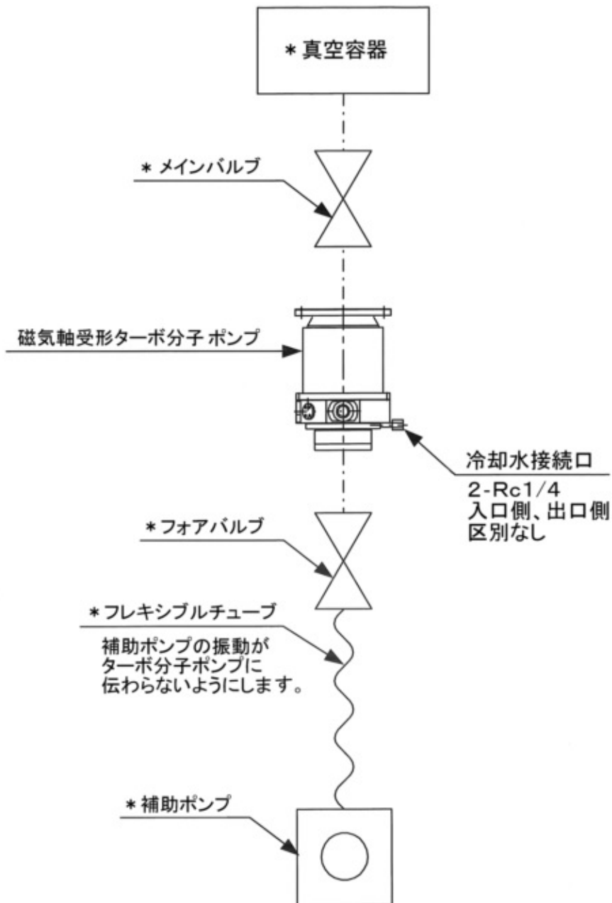
図 5-5 排気系の例
